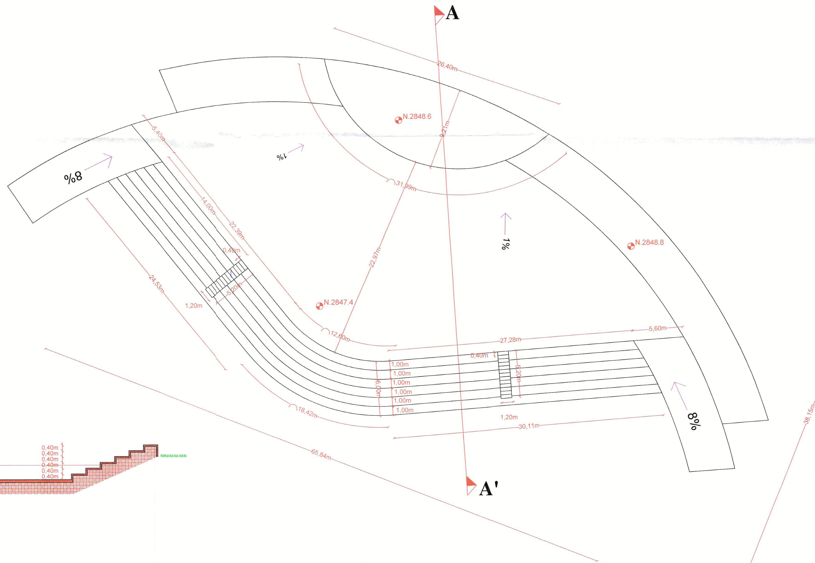
PLANTA ESCALA: 1:200
